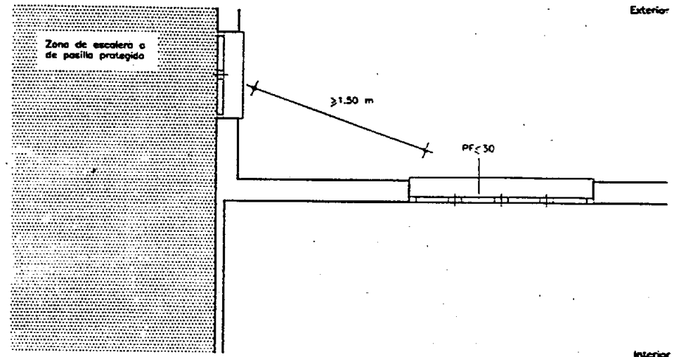
Planta
