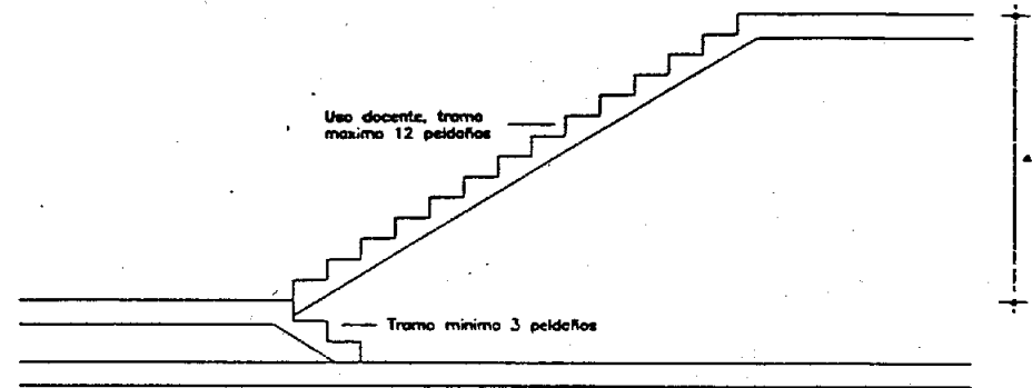
Sección
